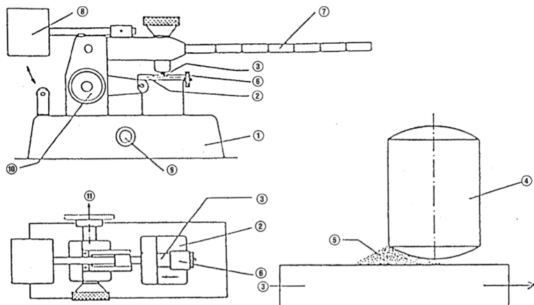
Fig. 5a Wrijvingstoestel; verticaal- en bovenaanzicht
