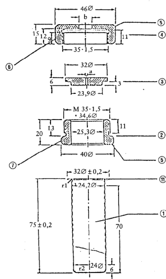
Fig. 1a Stalen buis en toebehoren
