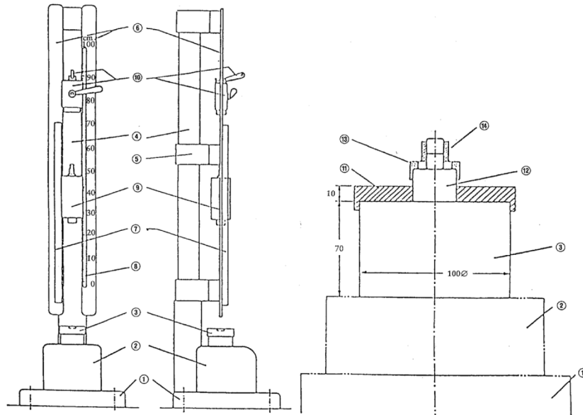
Fig. 4a Valhamer, voor- en zijaanzicht, overzicht
