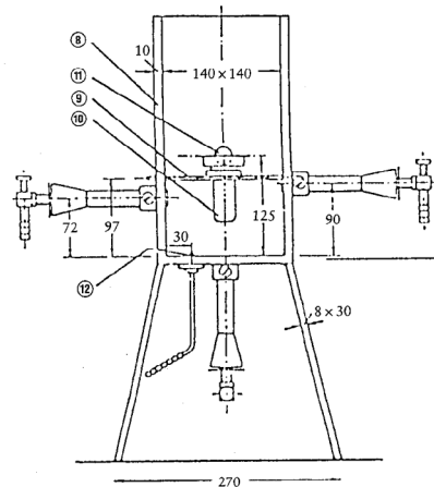
Fig. 1b Verwarmings- en beschermingstoestel
